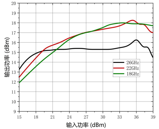
限幅电平
