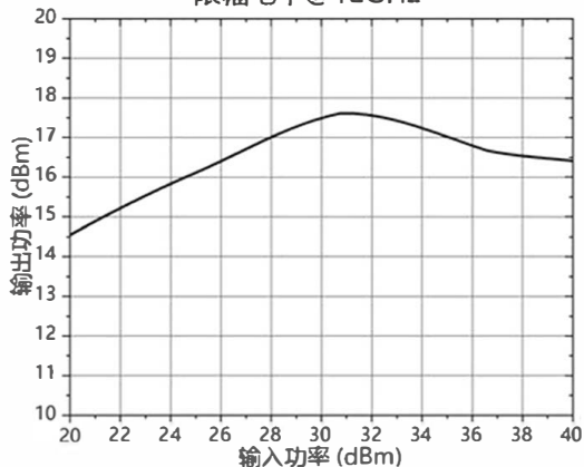
限幅电平@12GHz
