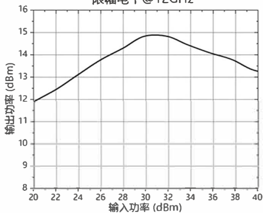
限幅电平@12GHz
