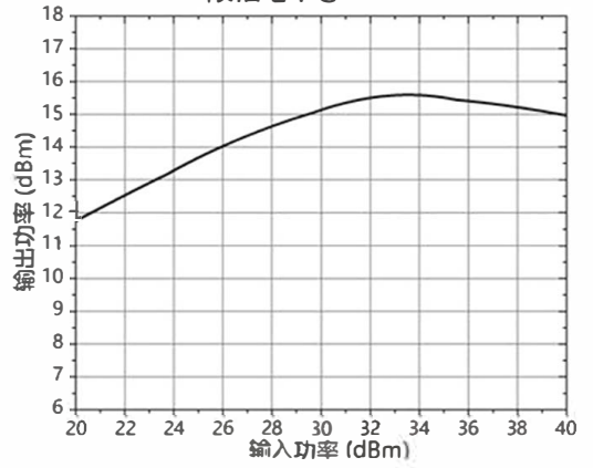
限幅电平@12GHz
